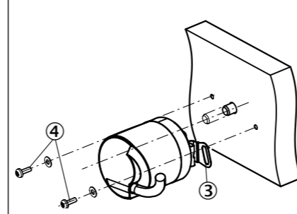
图2: 安装带定子联轴器(弹簧片)的 DBS36 盲孔空心轴型编码器
