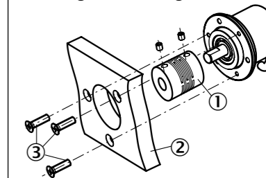
Abb. 6: Anbau DBS50 Klemmflansch über flanschseitige Gewindebohrungen
