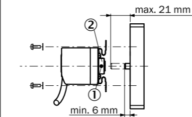
Abb. 1: Anbau DBS36 Aufsteckhohlwelle mit Drehmomentstütze
