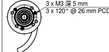
图1: 安装带定子联轴器(弹簧片)的 DBS36 盲孔空心轴型编码器
