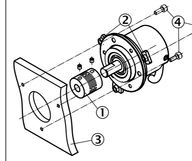
Abb. 8: Anbau DBS50 Klemmflansch mit Servoklammern
