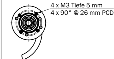
Klemmflansch Typ A
