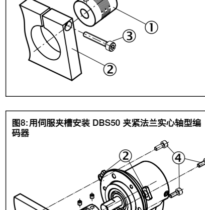
图8: 用伺服夹槽安装 DBS50 夹紧法兰实心轴型编码器
