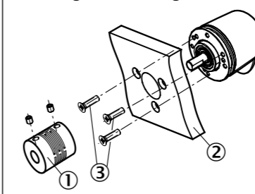
Klemmflansch Typ 0 (Standard Flansch)
