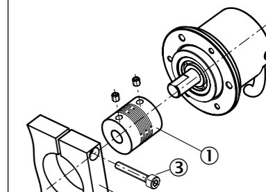
Abb. 7: Anbau DBS50 Klemmflansch über den Klemmansatz
