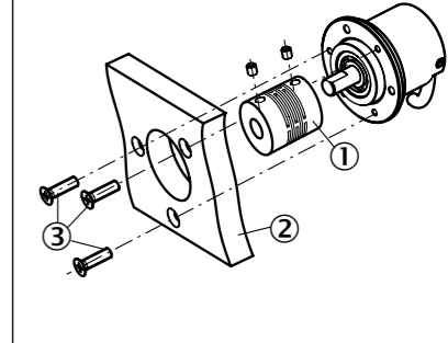
图6: 通过法兰一侧的螺纹孔安装 DBS50 夹紧法兰实心轴型编码器
