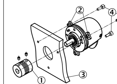
Abb. 5: Anbau DBS36 Klemmflansch mit Servoklammern
