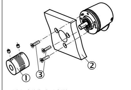
0型夹紧法兰(标准型法兰)
